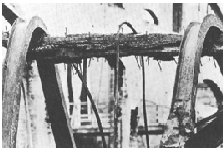
Figura 1: Mal desempeño de elementos de acero sin protección en un incendio.
