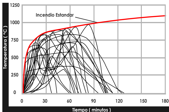
Figura 2: Esquema de obtención de la curva de incendio estándar.
