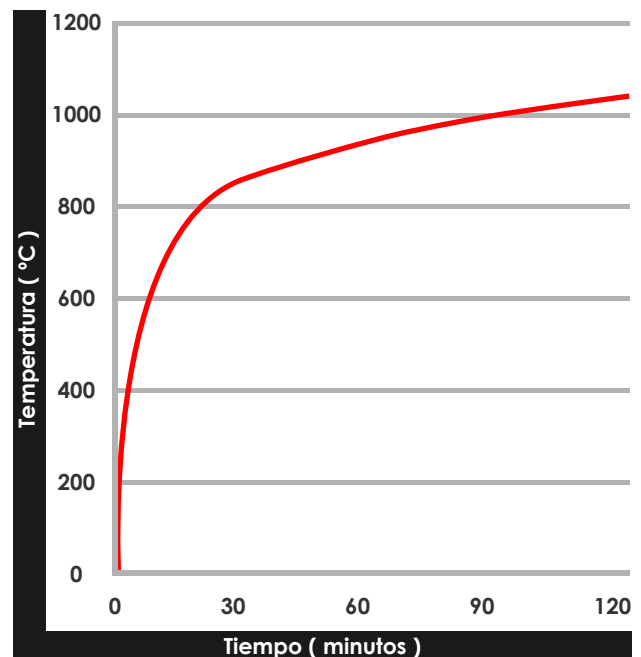
Curva de Incendio Estándar para Evaluación de Ensayo.
