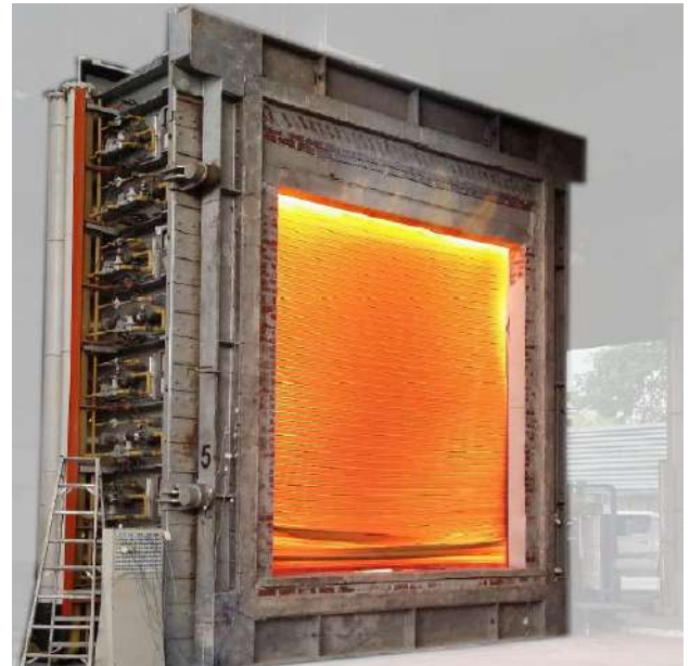
Horno de Ensayo de Resistencia al Fuego
